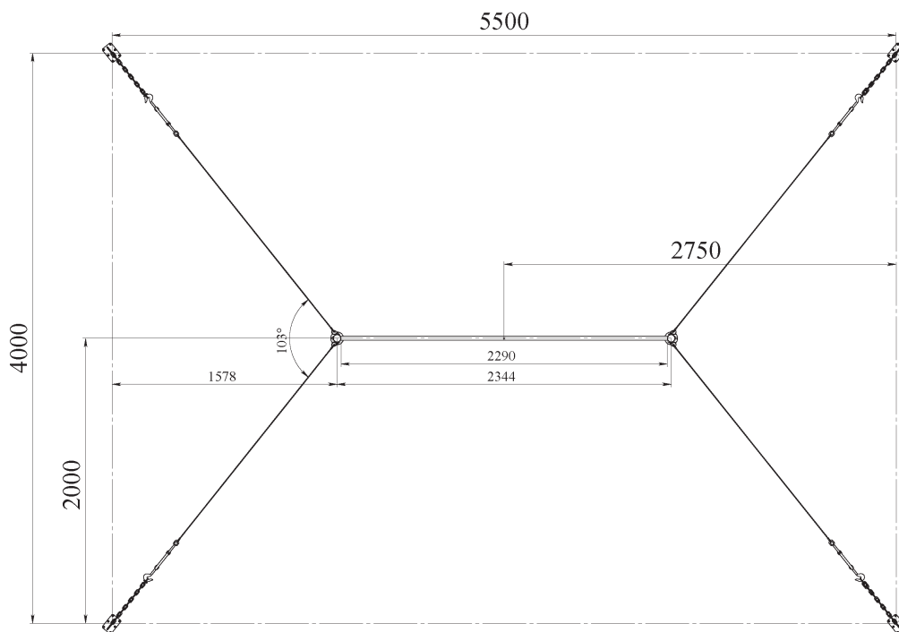
Схема установки перекладины универсальной на растяжках
